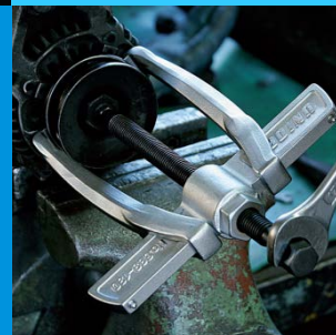
съёмники
